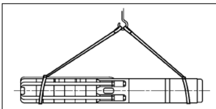
Схема строповки
